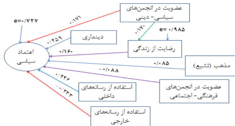
نمودار (۱) تحلیل مسیر بر اساس یافته‌های تحقیق
